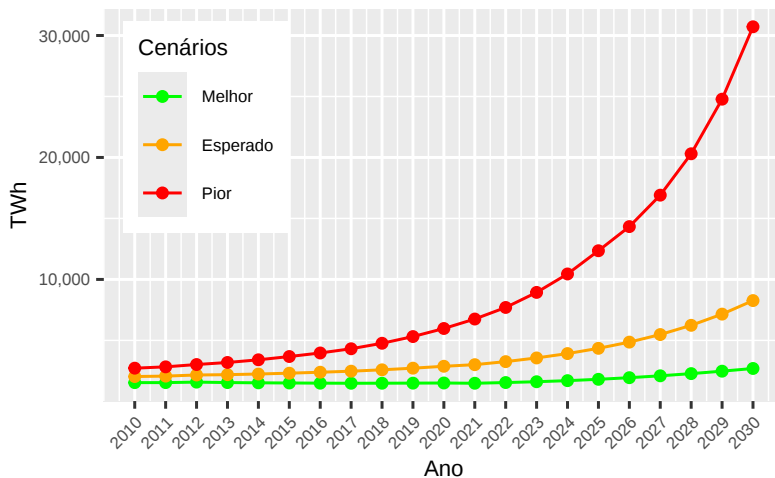
Figura 3.8: Consumo anual de energia em TWh por Tecnologias de Comunicação, estimado por Andrae e Edler (2015).
